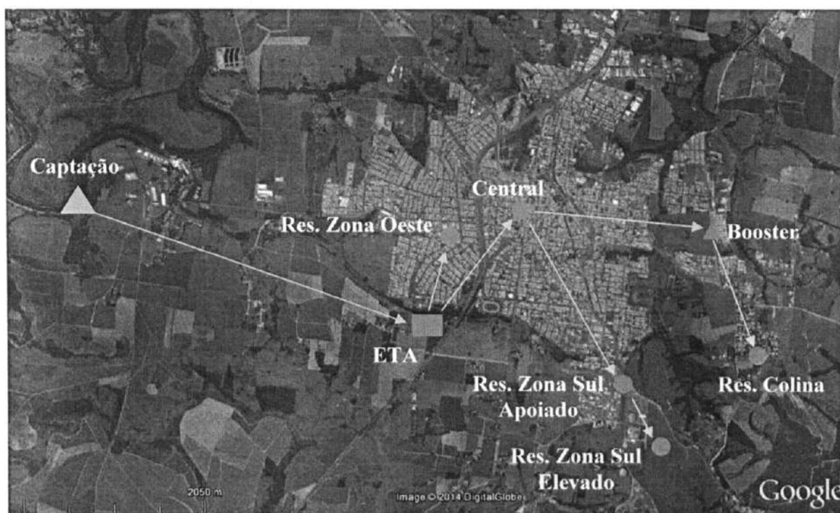
Figura 02. Localização das unidades do sistema de abastecimento de água do município de Cerquillo.
